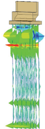
➔ 橋台基礎断面力
