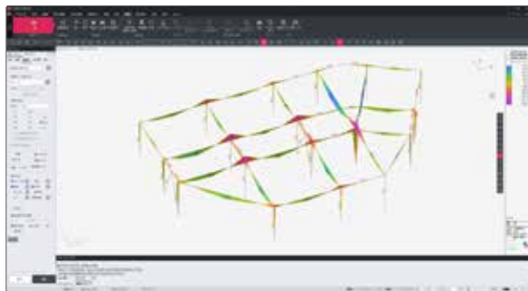
断面力図
