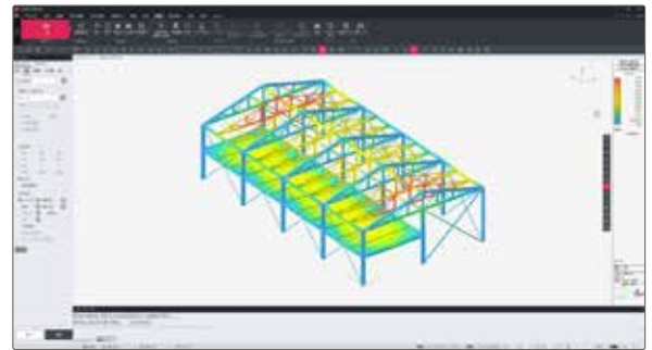
変位等高線
